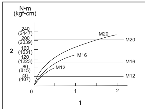
1. Tilspændingstid (sekunder) 2. Tilspændingsmoment
